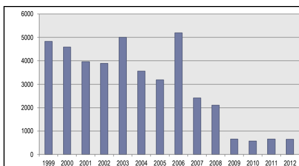
Rysunek 19. Emisja zanieczyszczeń pyłowych w Koninie w latach 1999-2012
